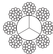
8x25 (12/6/6/1) AF FILLER
