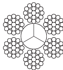
6x19 (12/6/1) AF 2 OPERACIONES
