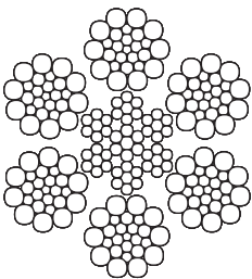
6X26 (10/5+5/5/1) AA CÓNDOR
